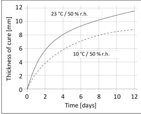
도표 1 : 경화 속도 SikaTack® DRIVE (60 min)
