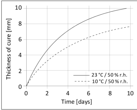
도표 1: Sikaflex®-515의 경화속도
